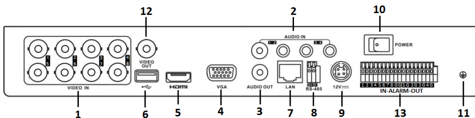
Obrázek 1–8 Zadní panel DS-7200HUHI-K
