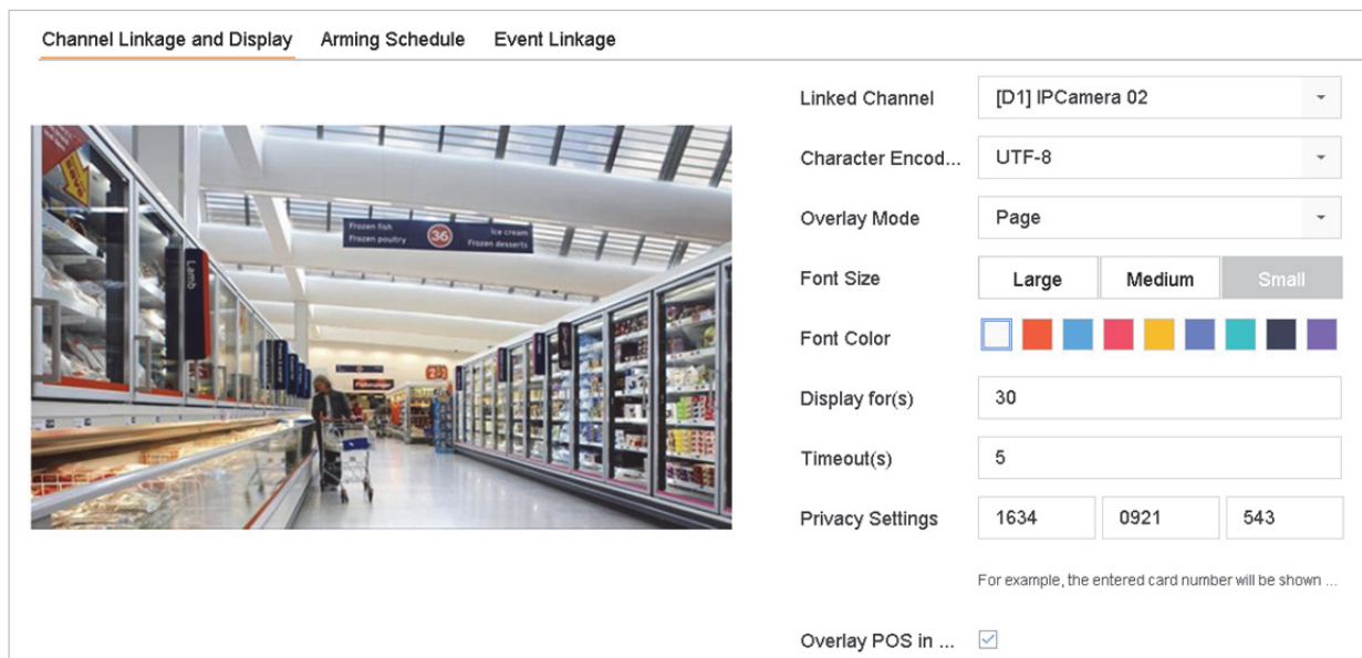
Obrázek 14–7 Nastavení překrytí znaky
