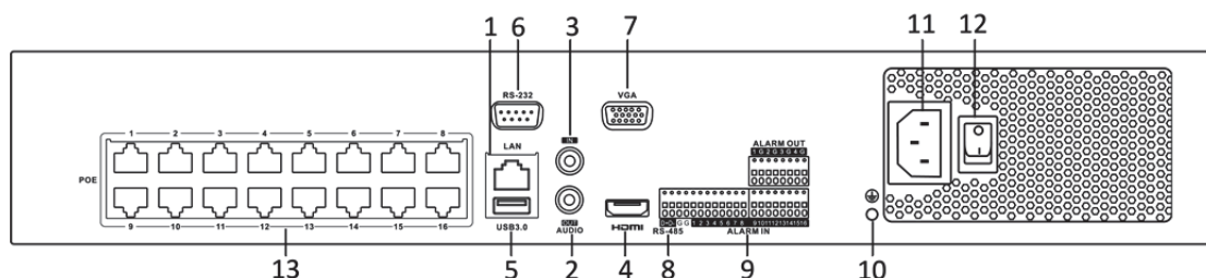
Obrázek 1–11 Řada DS-7700NI-I4/16P
